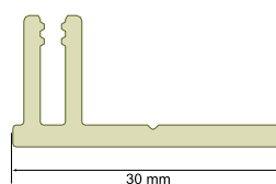
Eindprofiel (female) / 6023
