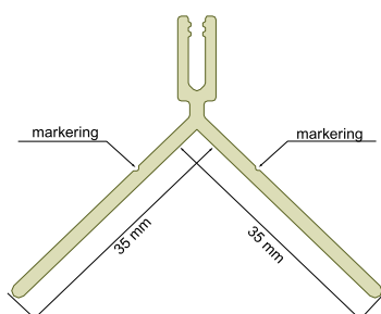
Hoekprofiel (female) / 6022
