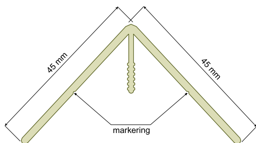
Hoekprofiel (male) / 6021
