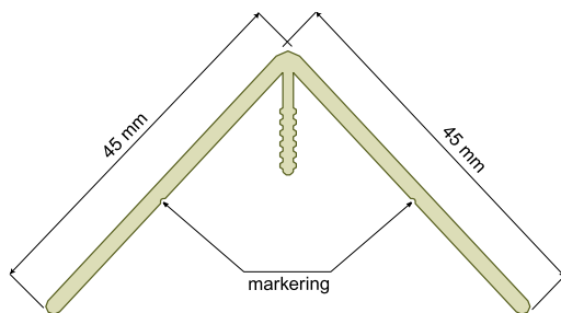
Hoekprofiel (male) / 6019
