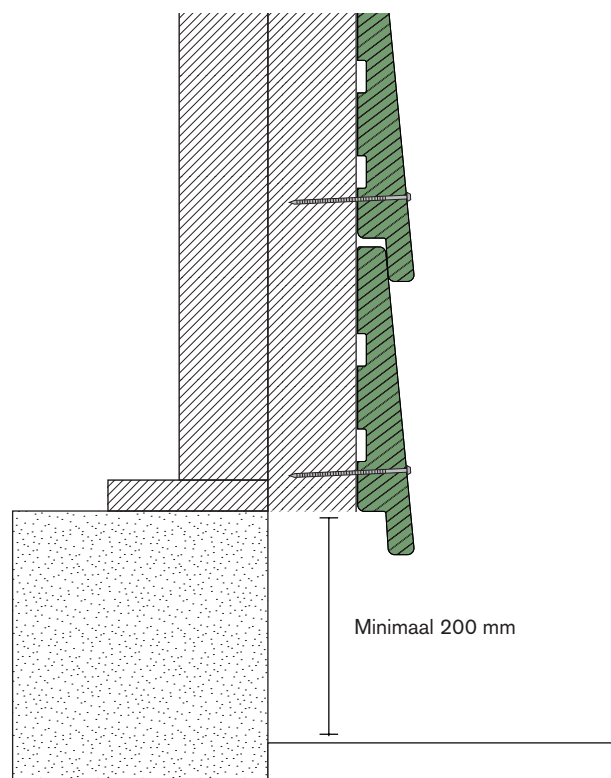
Doorsnede maaiveldhoogte
